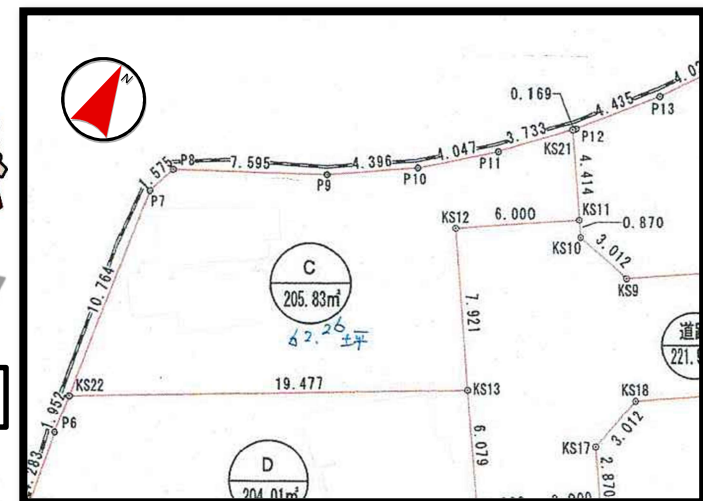
C号地 測量図
